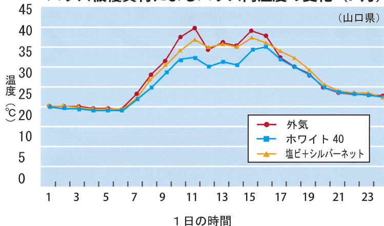
ハウス被覆資材によるハウス内温度の変化 (7月)
