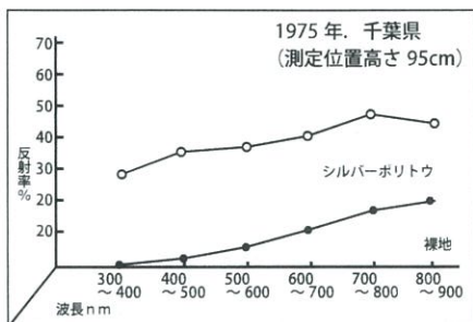
波長別畑内反射率
