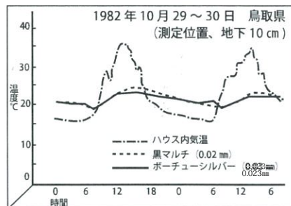
ボーチューシルバーの地温変化
