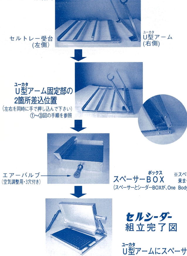
セルホルダー分解図
